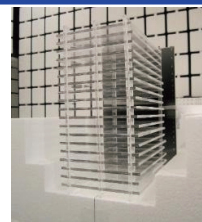
実測写真(水平方向) シミュレーション構造(垂直方向) ホーンアンテナと誘電体材料
