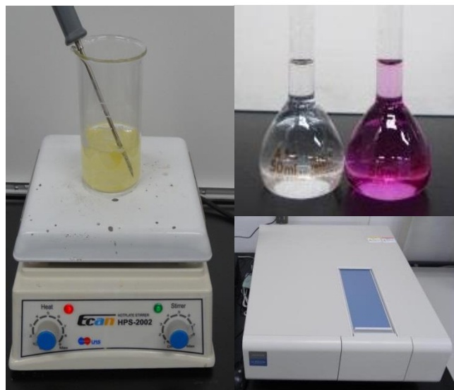
図1. 六価クロム抽出工程（左）、ジフェニルカルバジドによる呈色（右上）、吸光度計による測定（右下）
